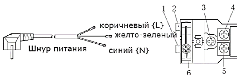
Клеммная коробка
